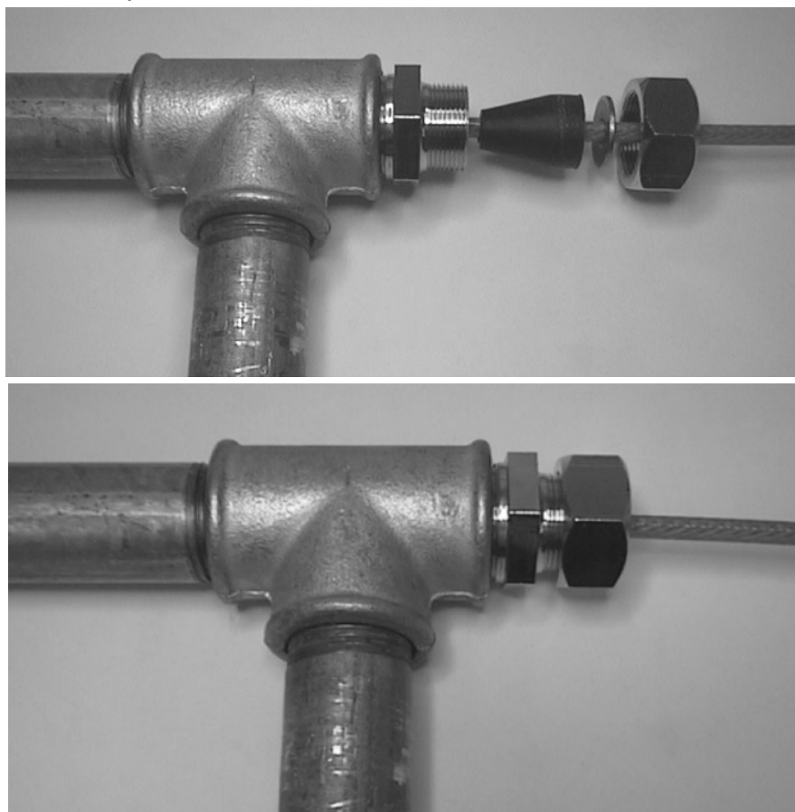
Рис.3. Технология установки зажимной муфты на трубопровод.
