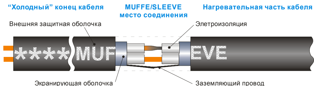
Рис.1. Конструкция безмуфтового соединения двухжильного нагревательного кабеля Hemstedt BR-IM
