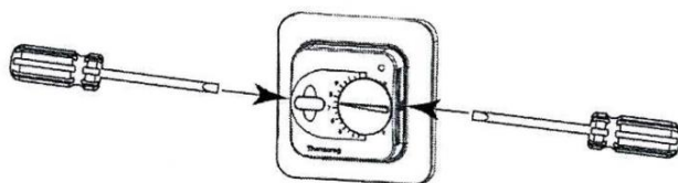
Рис. 1 Снятие передней панели
