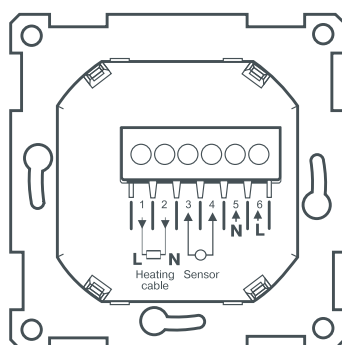
Рис. 2 Соединения термостата
